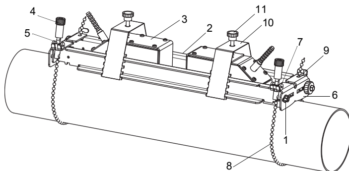
Рис. 6.11: Портативное монтажное крепление с цепями
