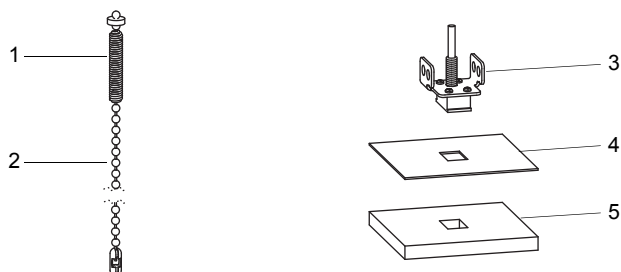
Рис. 6.16: Датчик температуры
