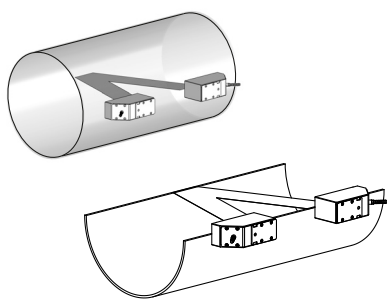
Рис. 3.9: 2 прохода звука в одной плоскости
