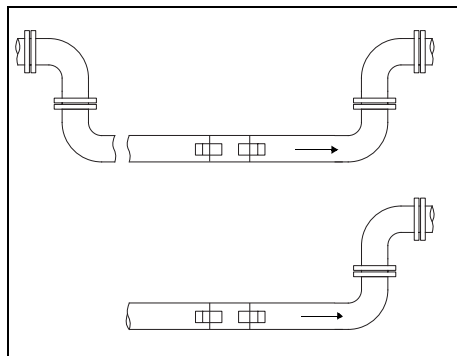
Рис. 3.14: Рекомендуемое размещение датчиков
