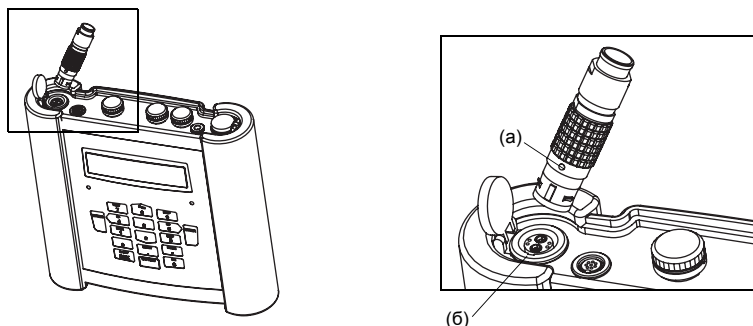
Рис. 7.2: Подключение датчиков
