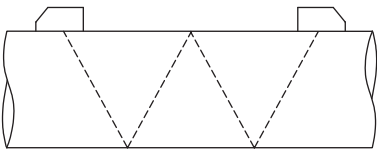
Рис. 3.7: Режим отражения с 1-м лучом и 4-мя проходами звука
