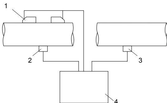
Рис. 21.2: Измерение теплового потока при измерении расхода на подающей трубе
