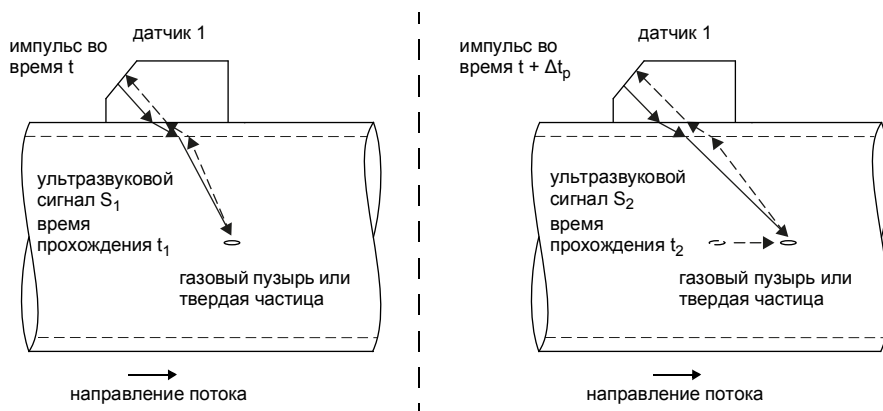
Рис. 3.4: Измерение скорости потока в режиме NoiseTrek
