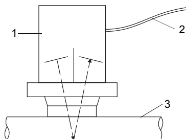
Рис. 20.1: Принцип измерения
