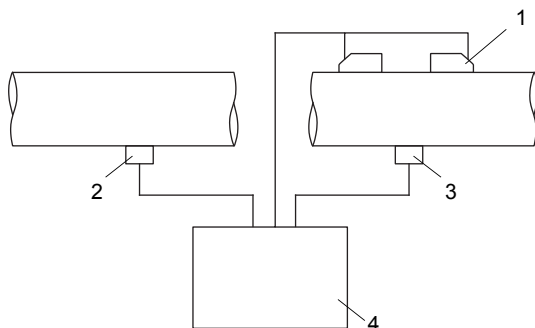
Рис. 21.1: Измерение теплового потока при измерении расхода на обратной трубе
