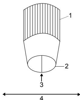
Рис. 20.2: Установка датчика толщины стенки
